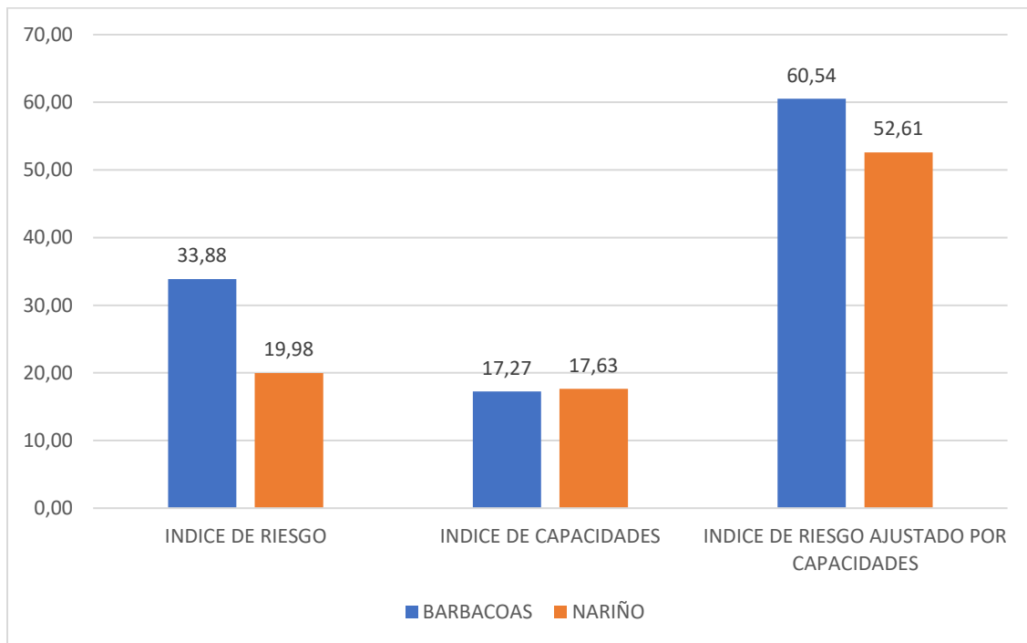
Gráfica 49. Municipio de Barbacoas, Índices de riesgo de Desastres 2018.
